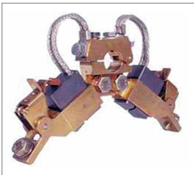
Borsthållare för elmotorer
